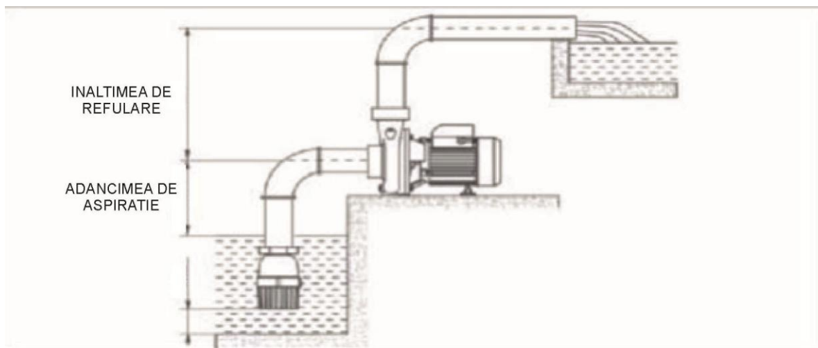
Schema instalarii
