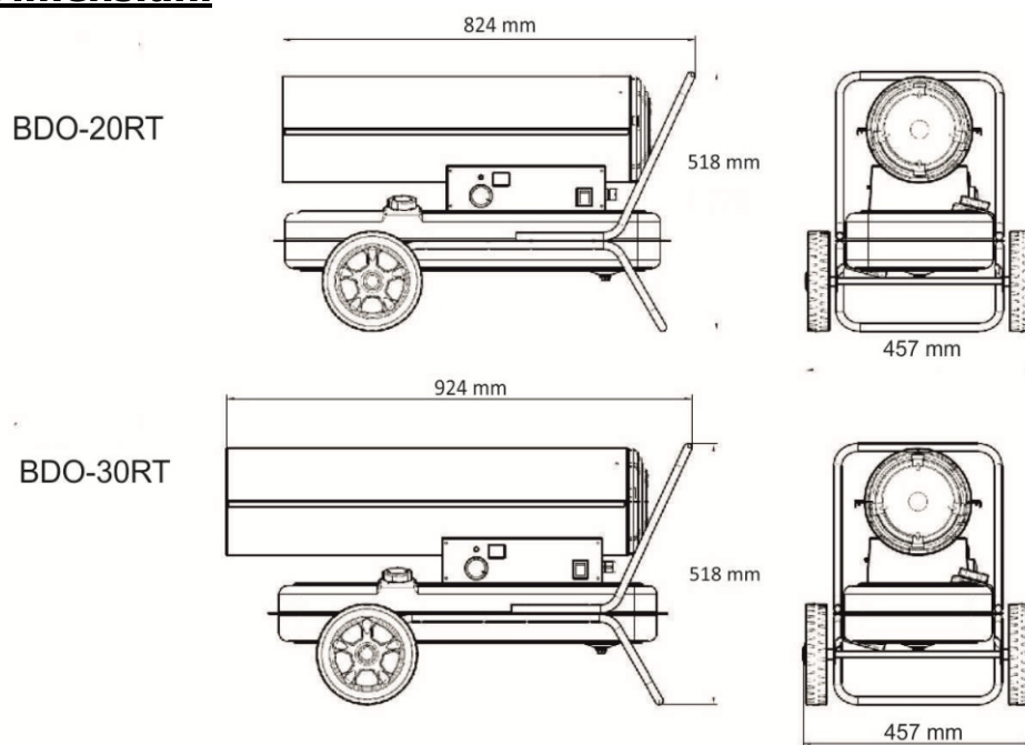
Figura 2. Dimensiunile produsului
